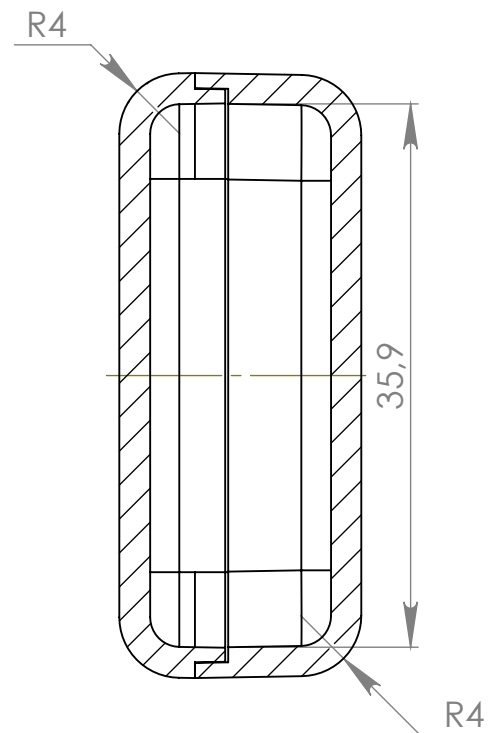
PRZEKRÓJ B-B SKALA 2 : 1
